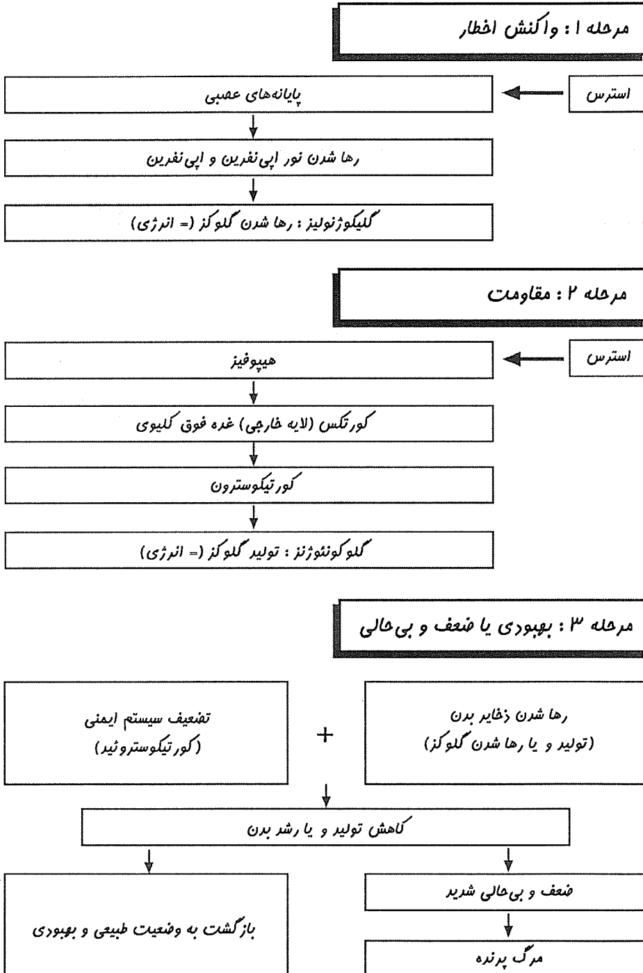
شکل ۱۳- مکانیسم استرس
